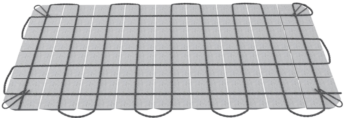
Рисунок Б.4 - Схема расположения угловых соединительных петель ПБЗГУ модели 105
