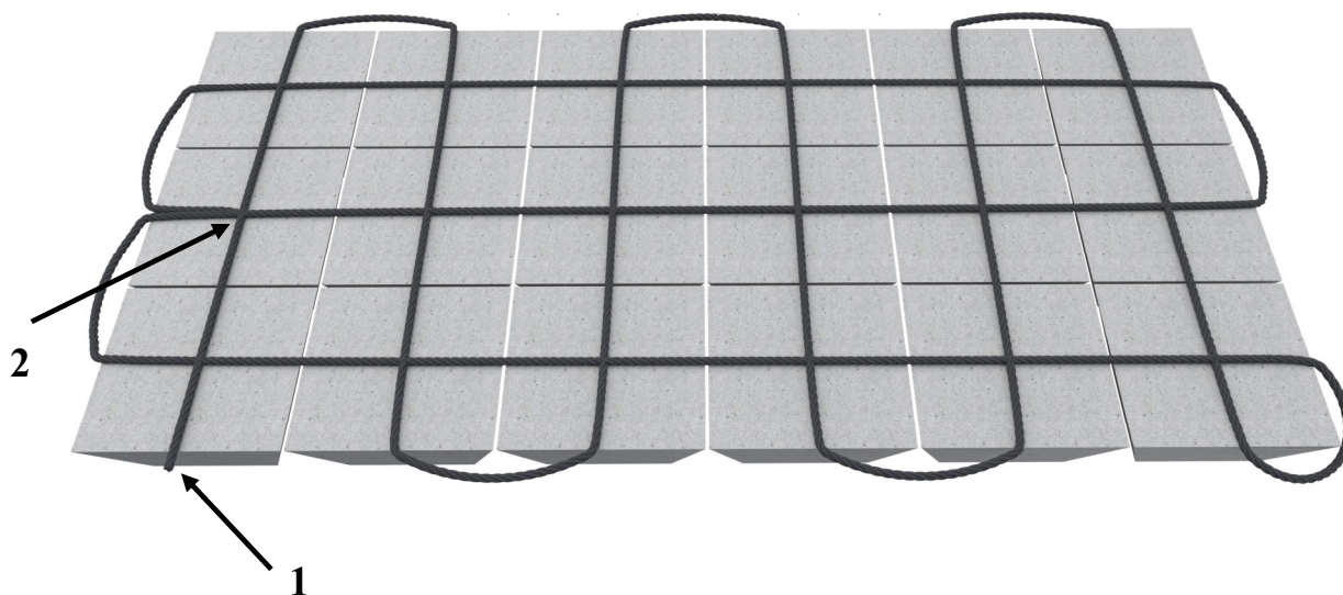
Рисунок Б.2 – Укладка соединительного арматурного каната в формообразующую оснастку плиты модели 712 1 – начало укладки каната, 2 – конец укладки каната
