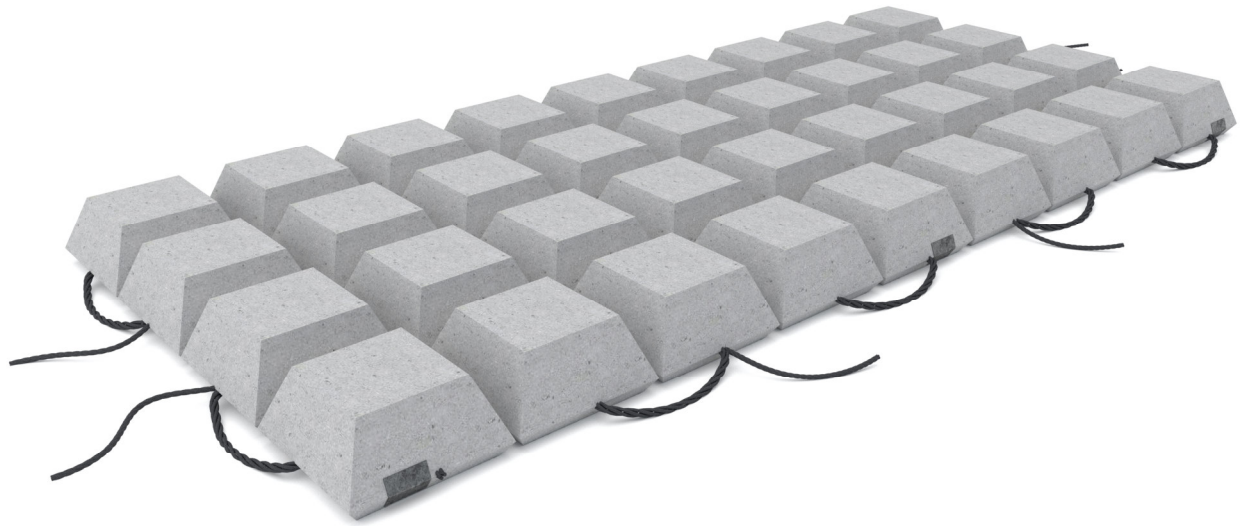
Рисунок А.3 – Конструкция ПБЗГУ модели № 405
