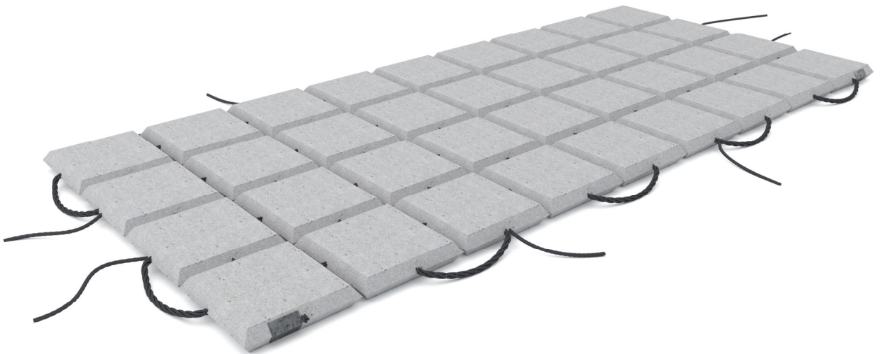
Рисунок А.2 – Конструкция ПБЗГУ модели № 202
