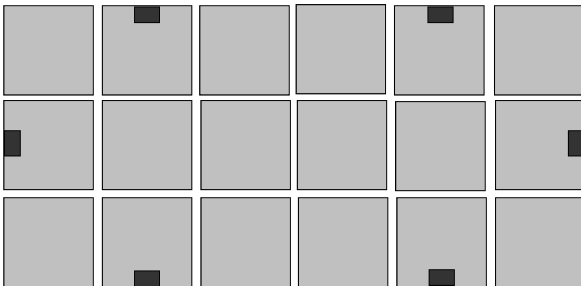
Рисунок Б.8 – Рисунок расположения закладных деталей при бетонировании ПБЗГУ модели 712
