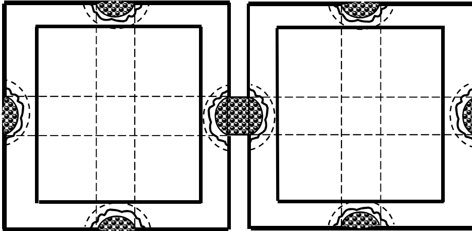
Рисунок Г.1 – Технологическая выемка в месте выхода арматурного каната из бетонного блока
