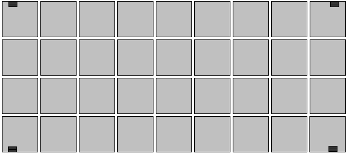
Рисунок Б.5 – Рисунок расположения закладных деталей при бетонировании ПБЗГУ модели 202
