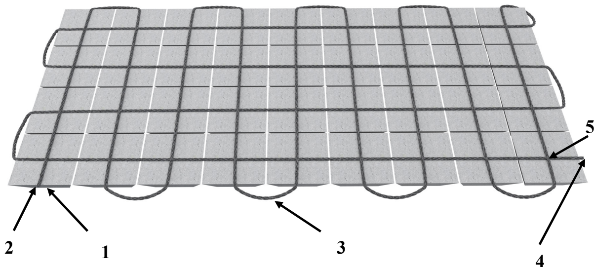
Рисунок Б.1 – Укладка соединительного арматурного каната в формообразующую оснастку плит моделей 105, 202, 405
