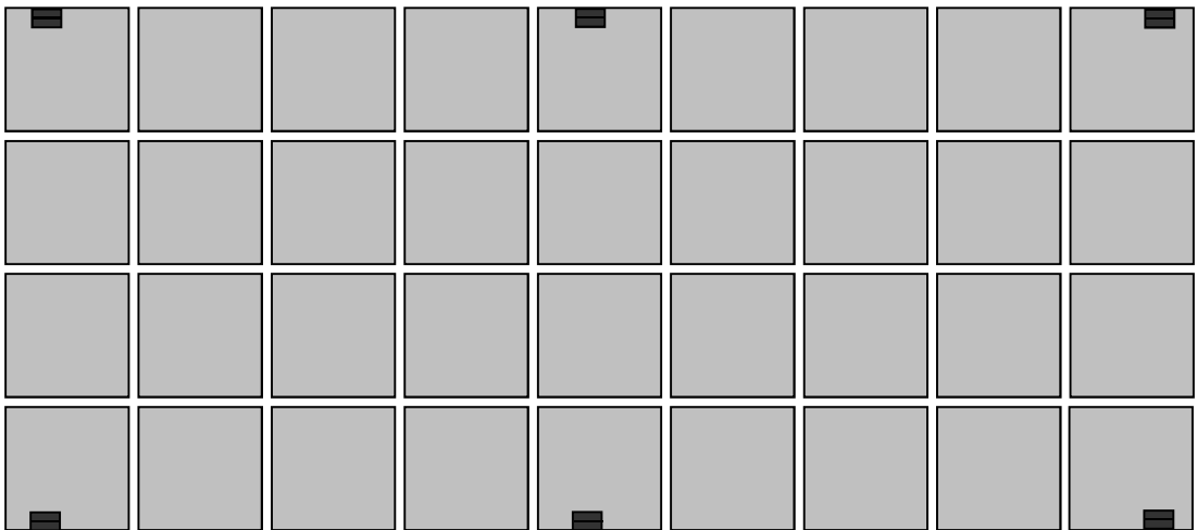
Рисунок Б.6 – Рисунок расположения закладных деталей при бетонировании ПБЗГУ моделей 105 и 405
